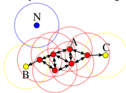
FIGURA 9 NELLA FIGURA, \text{minPts}=3 , A È UN CORE POINT, B E C SONO DENSITY-REACHABLE POINTS MENTRE N È UN NOISE POINT 70
