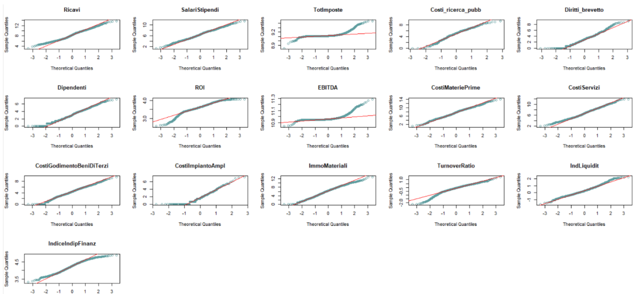
FIGURA 15 QQ-PLOT NORMALI DELLE IMPRESE DI FILIERA, DOPO TRASFORMAZIONE LOGARITMICA E RIMOZIONE DEGLI OUTLIER
