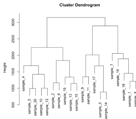
FIGURA 5 ESEMPIO DI DENDROGRAMMA 53
