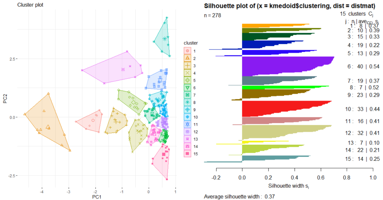
FIGURA 29 RISULTATI DEL CLUSTERING KMEDOIDS E SILHOUETTE MEDIA DI CIASCUN CLUSTER La silhouette media è del 37%. Lo stesso indice consente di misurare la qualità di ciascun gruppo.
