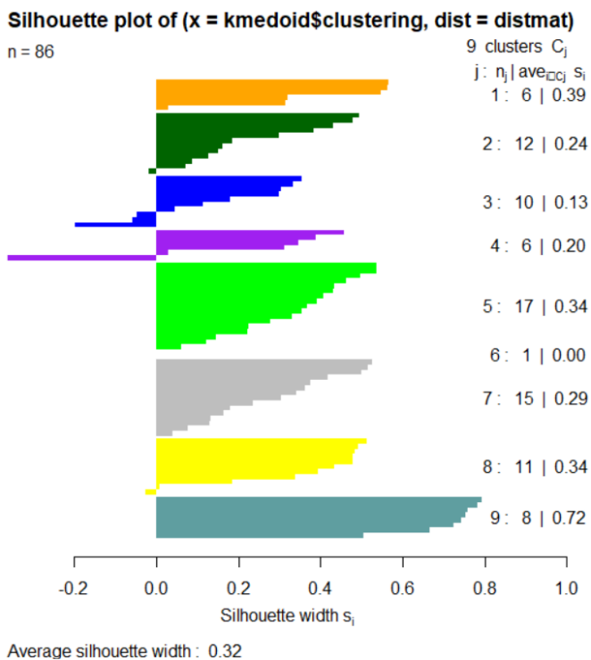
FIGURA 47 SILHOUETTE DEI CLUSTER DELLE PROVINCE
