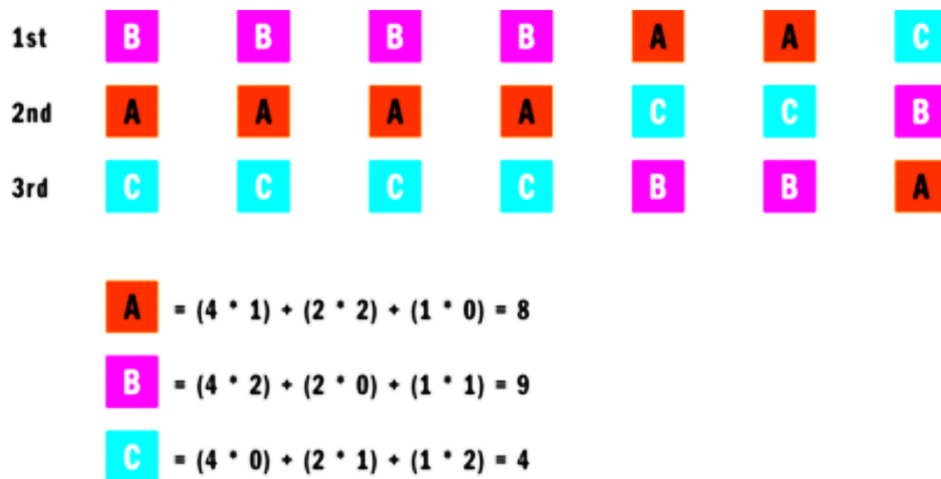
FIGURA 10 ESEMPIO DI CALCOLO DI TRE PUNTEGGI BORDA IN UNA COMPETIZIONE CON TRE CONCORRENTI E SETTE CONFRONTI 83
