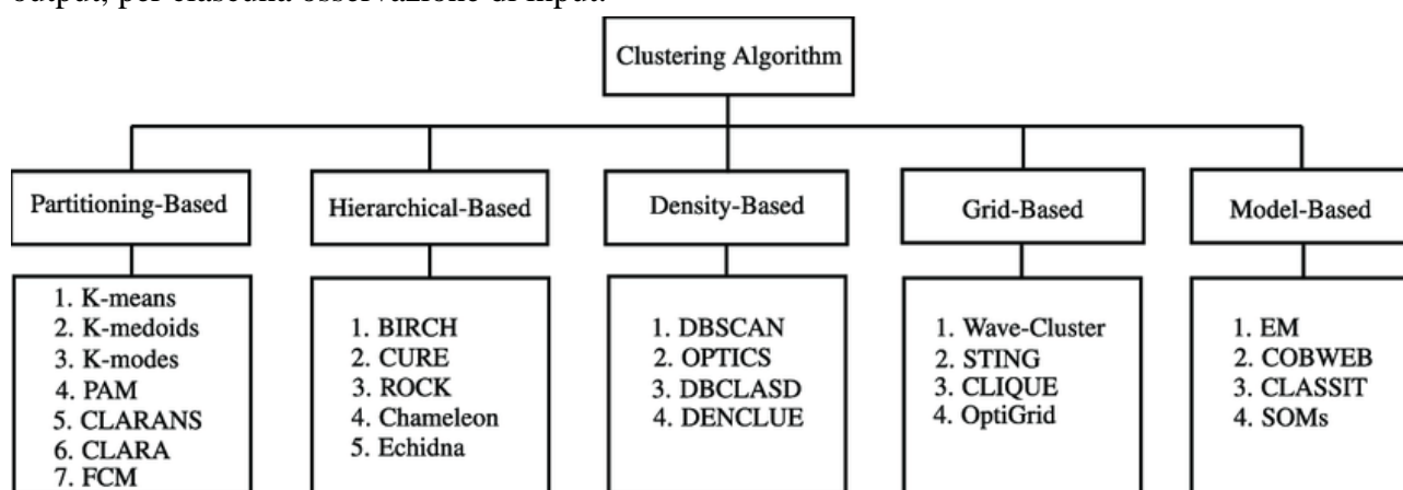
FIGURA 2 CLASSIFICAZIONE DEGLI ALGORITMI DI CLUSTERING 38
