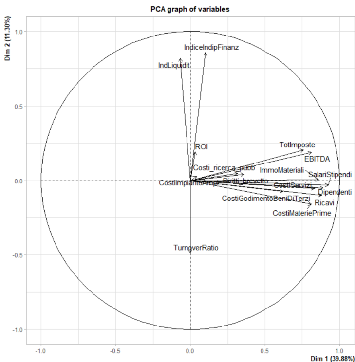
FIGURA 20 BIPLLOT: VARIABILI CON DIREZIONI PARALLELE SONO RECIPROCAMENTE CORRELATE, VARIABILI CON DIREZIONI PERPENDICOLARI PRESENTANO CORRELAZIONE NULLA
