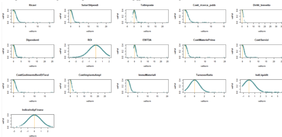
FIGURA 12 PDF NORMALI DELLE VARIABILI NEI DATI GREZZI SULLE IMPRESE DELLA FILIERA
