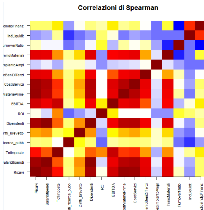
FIGURA 16 COEFFICIENTI DI SPEARMAN: COLORI SCURI IMPLICANO ALTA CORRELAZIONE Correlazioni di Spearman
