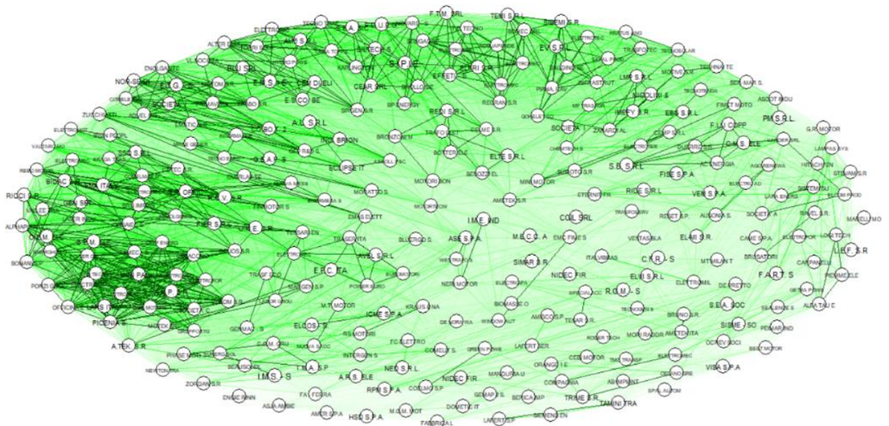
FIGURA 24 MATRICE DELLE DISTANZE CON DISTANZA EUCLIDEA SOTTO FORMA DI GRAFO: ARCHI CORTI E SCURI IMPLICANO FORTE SOMIGLIANZA TRA OGNI COPPIA DI OSSERVAZIONI
